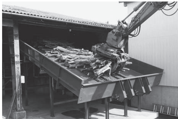
原木投入チェーンライブデッキ
